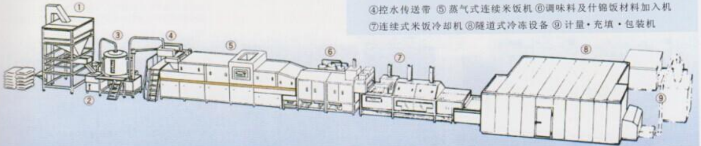
冷冻米饭生产线系统流程图
